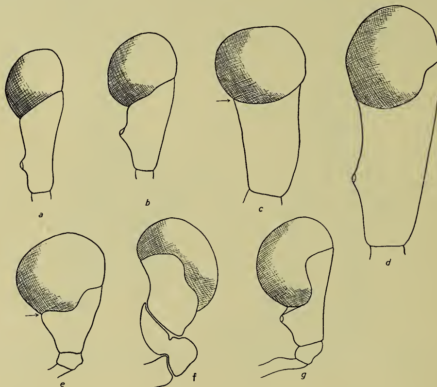
TEXT-FIG. 12.—Ocular peduncle of (a) Hepomadus tener ; (b) Hemipenæus crassipes ; (c) Plesio-penæus edwardisianus ; (d) P. armatus ; (e) Aristeomorpha foliacea ; (f) Parapenæus fissurus ; (g) Aristeus alcocki . The arrow indicates the position of the ocular tubercle.
